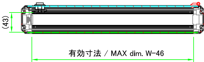
A-A ( 1 : 5 )
